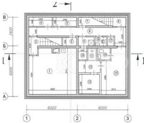
Экспликация помещений
