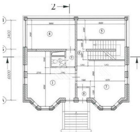
Экспликация помещений
